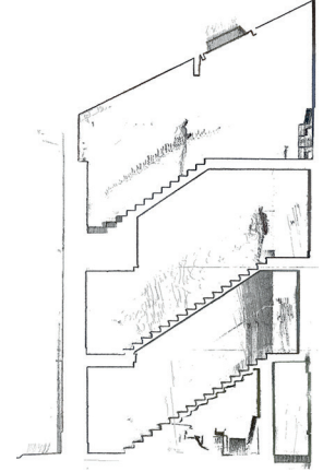
COUPE VERTICALE
